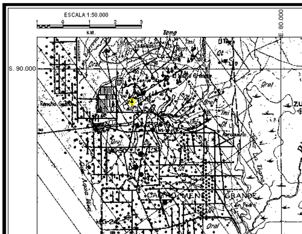
Tomado de: Geología de Superficie de la Creole Petroleum Corporation, Hoja E-4-A, 1960.
